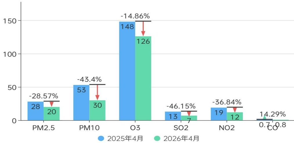
图1 我市2025年4月与2026年4月空气质量对比图
